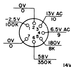
XTAL OSC V207 6BH6
